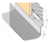
Solins Bavettes Plomb Arrêt d'Enduit
